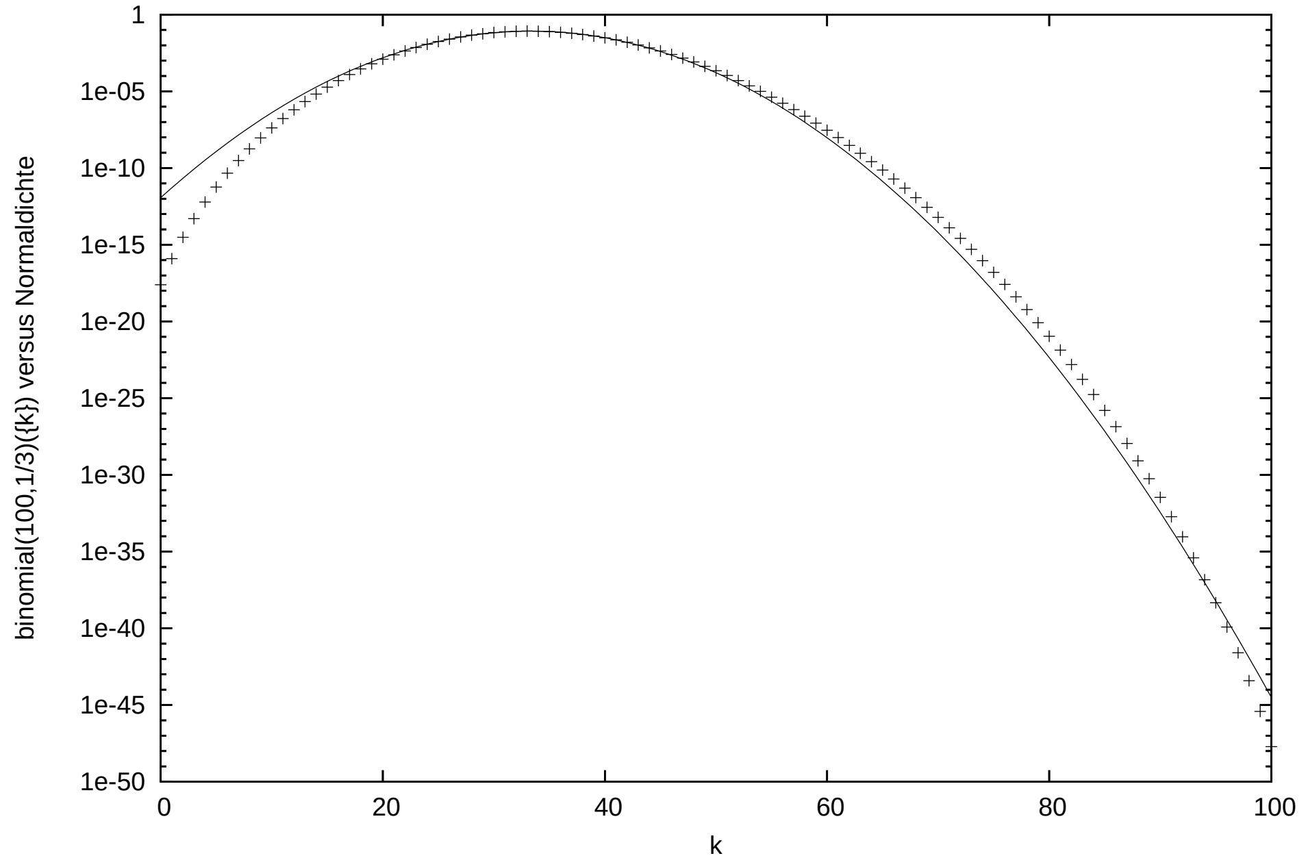
Binomial-Zaehldichte versus Normaldichte (Logarithmisch dargestellt)
