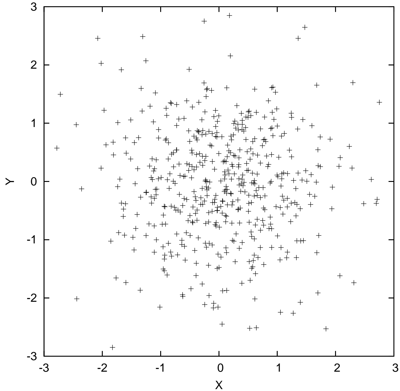
500 iid normalverteilte Datenpunkte: Korrelation r=0
