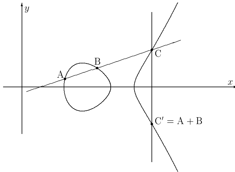
Bild 3. Addition auf elliptischen Kurven
