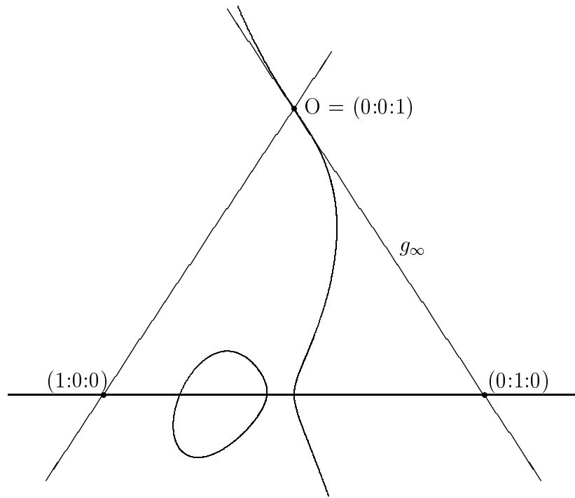
Bild 2. Elliptische Kurve in der projektiven Ebene
