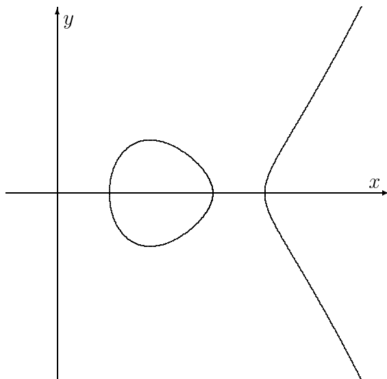
Bild 1. Elliptische Kurve y^2 = (x - c_1)(x - c_2)(x - c_3)
